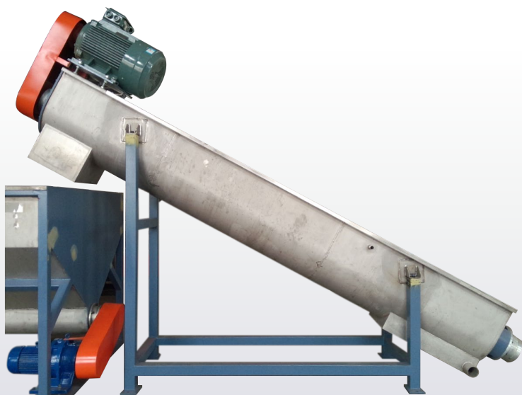
Шнековый конвейер моечного комплекса
