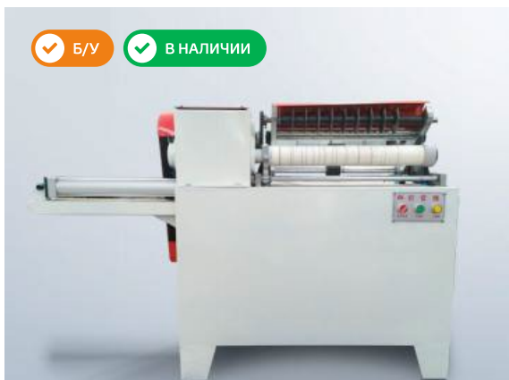
УСТРОЙСТВО АВТОМАТИЧЕСКОЕ РЕЗКИ ШПУЛЬ, МОДЕЛЬ LD-P1300
